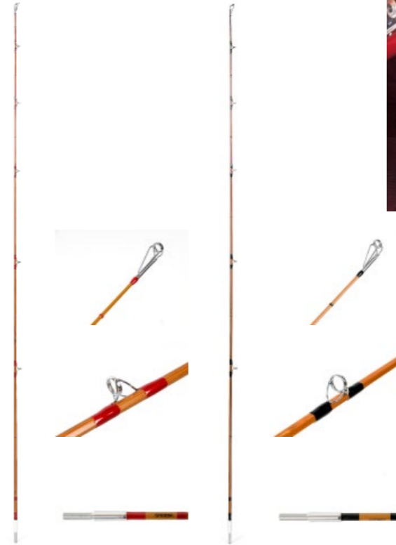
26-668-01 (88159A) バットフェルルVer.2(A) 本体寸法:5ft(1/8~5/8oz) 竹 アルミ/漆塗装(グリップ別売) (バットフェルルシルバー・ローズ)
